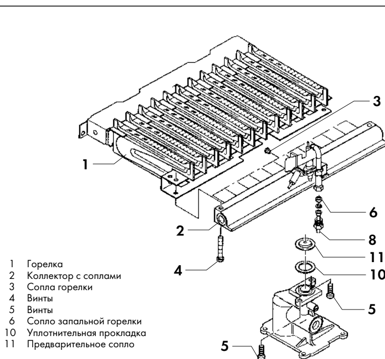
Рис. 20: Перенастройка на другой вид газа
