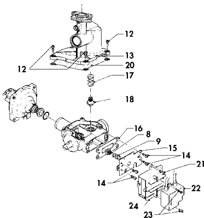
Рис. 20.1: Перенастройка на другой вид газа
