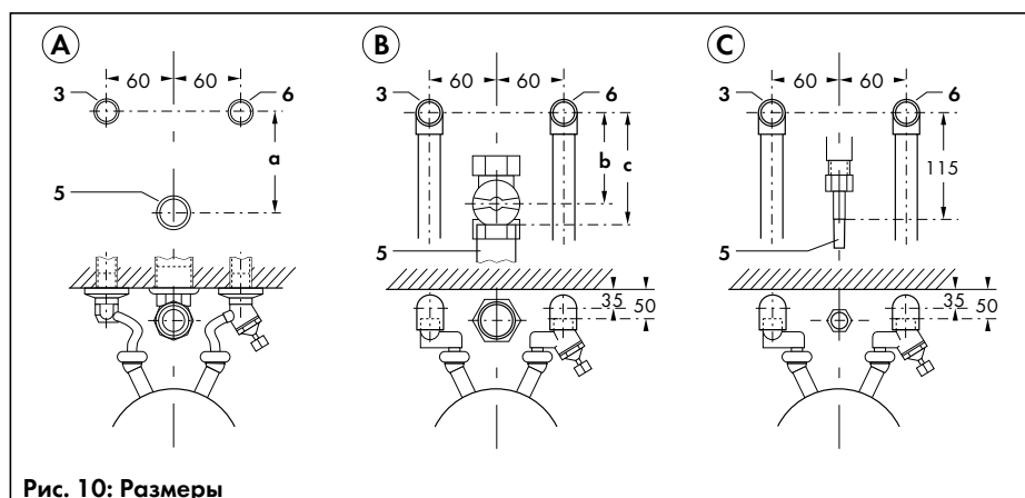
Рис. 10: Размеры
