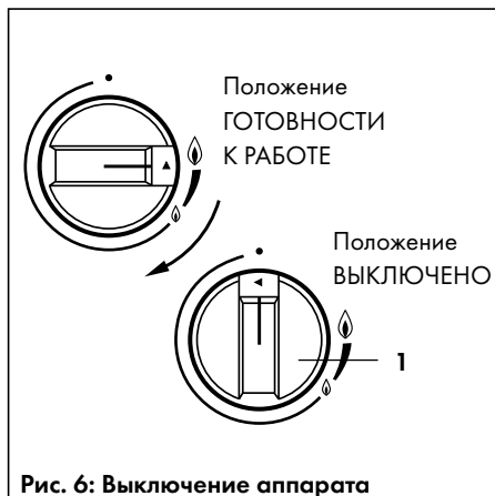
Рис. 6: Выключение аппарата
