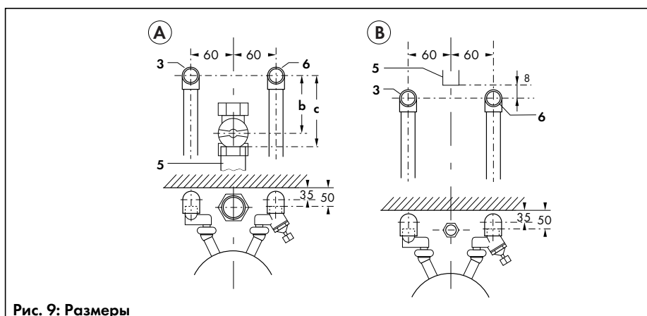
Рис. 9: Размеры
