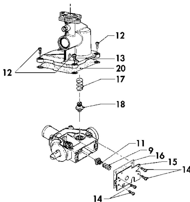
Рис. 18.1: Перенастройка на другой вид газа
