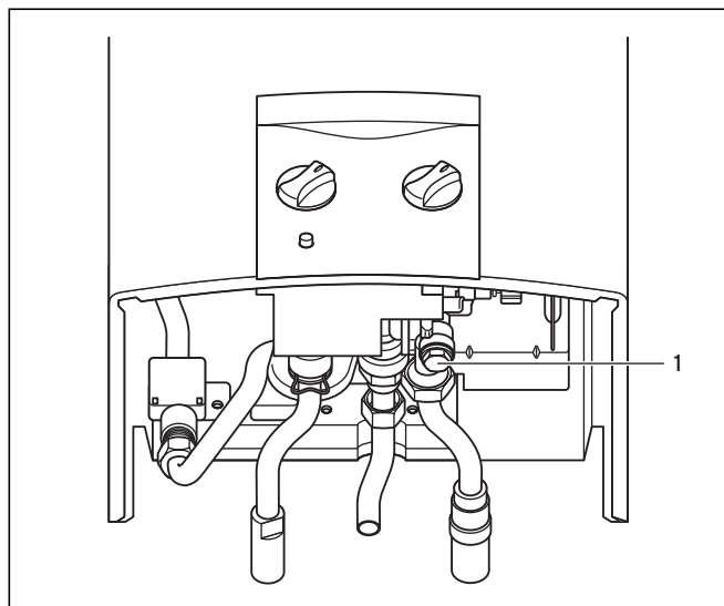
Рис. 4.8 Слив воды
