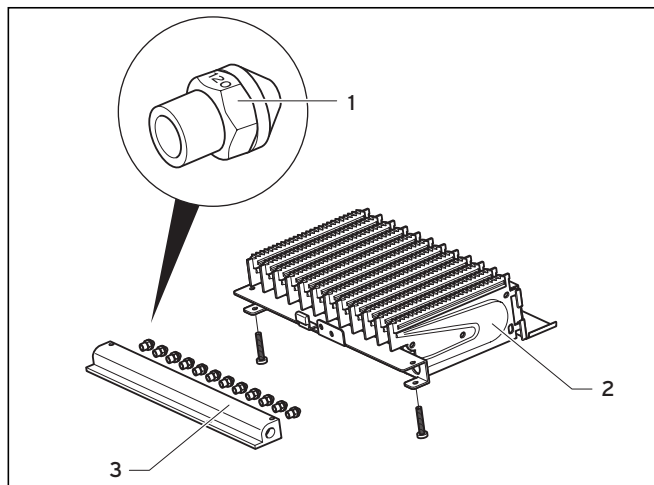
Рис. 6.6 Маркировка сопла
