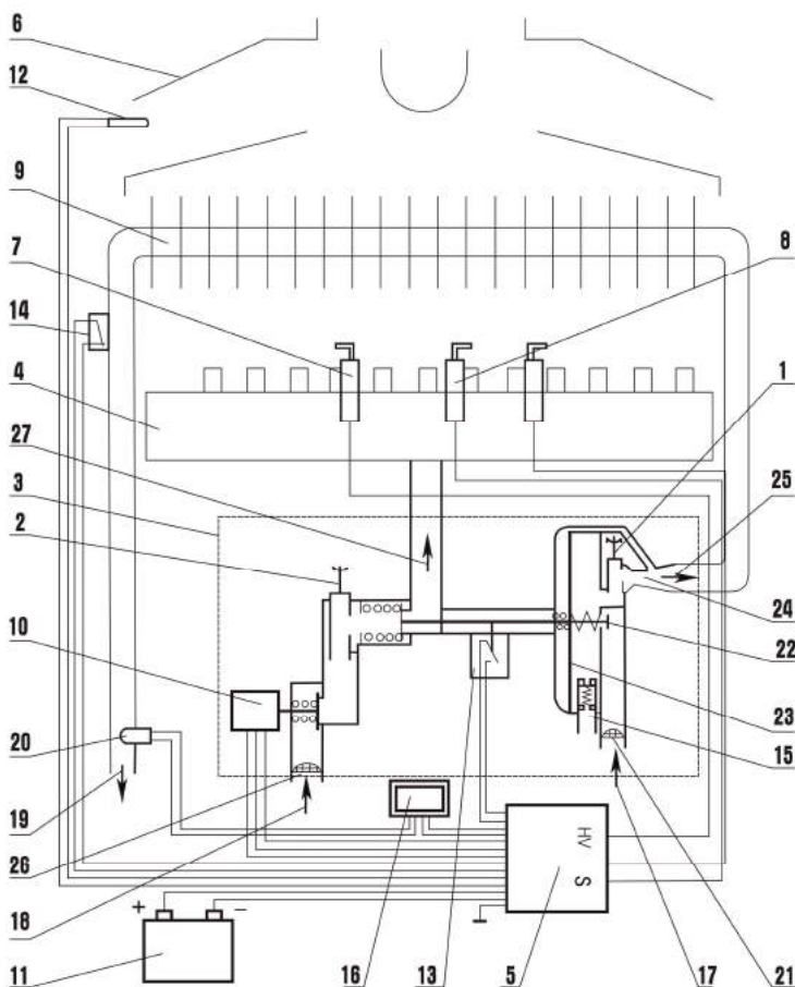
Рис. 4.3 – Функциональная схема водонагревателя
