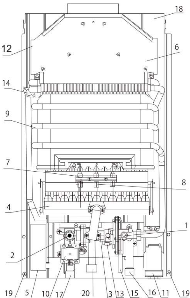
Рис. 4.2 – Внешний вид водонагревателя без облицовки
