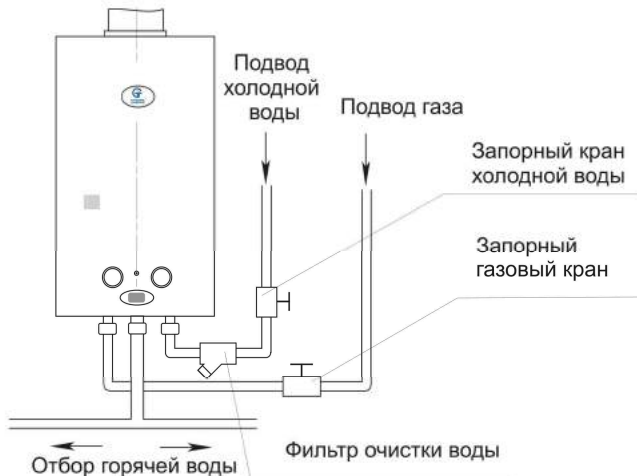
Рис. 5.5 – Схема подключения водонагревателя
