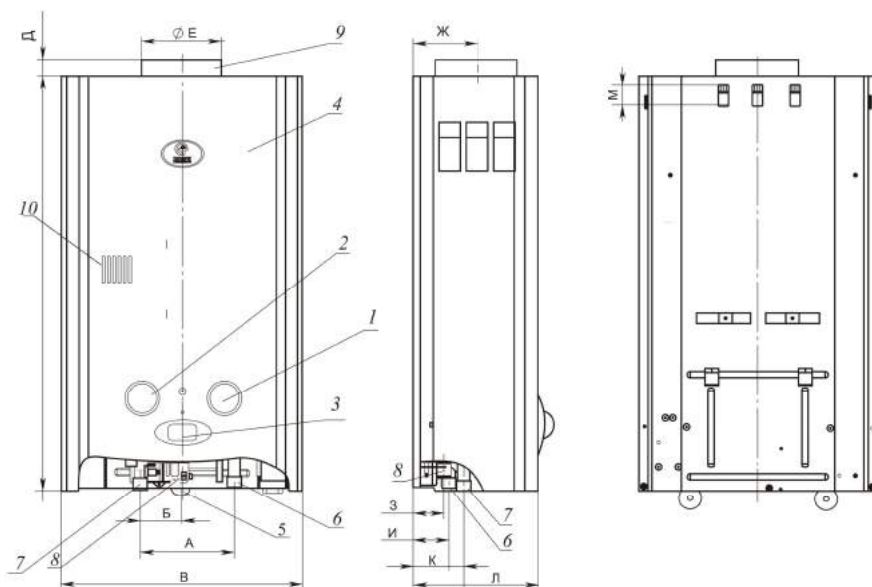
Рис. 4.1 – Внешний вид, габаритные размеры и присоединительные размеры аппарата (ДА)
