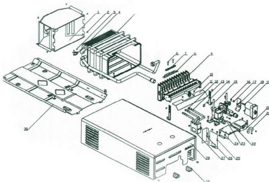
Рис.7.15 – Запасные части водонагревателя
