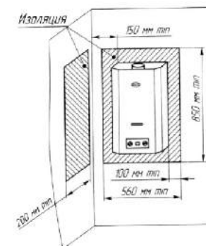
Рисунок 6. Установка аппарата на трудно-сгораемых стенках
