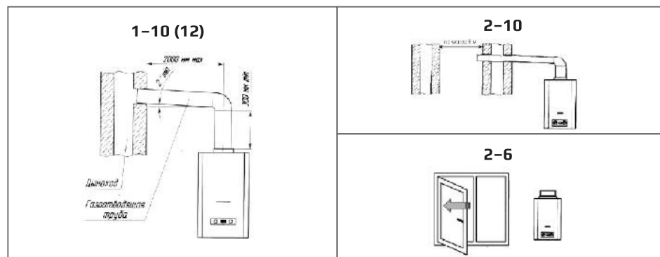
Рисунок 8. Подключение аппаратов к дымоходу
