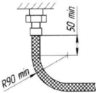
Рисунок 7. Требования к изгибам гибких шлангов
