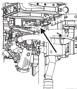
Рис 11 Точка измерения давления перед форсункой
