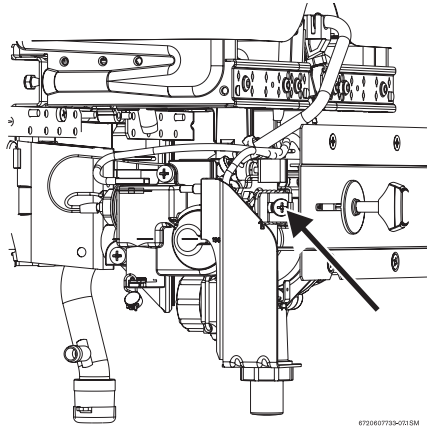
Рис 13 Вит регулировки мин. расхода газа
