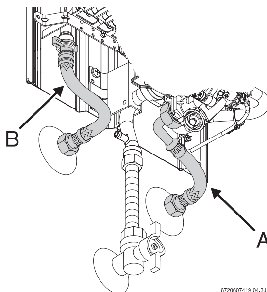
Рис 4 Подключение водопровода
