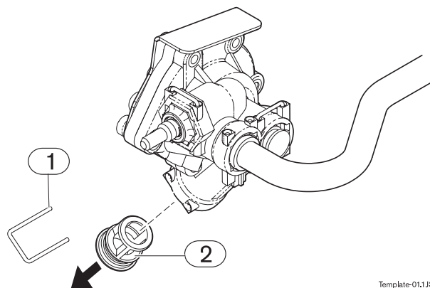
Рис 15 Опорожнение прибора
