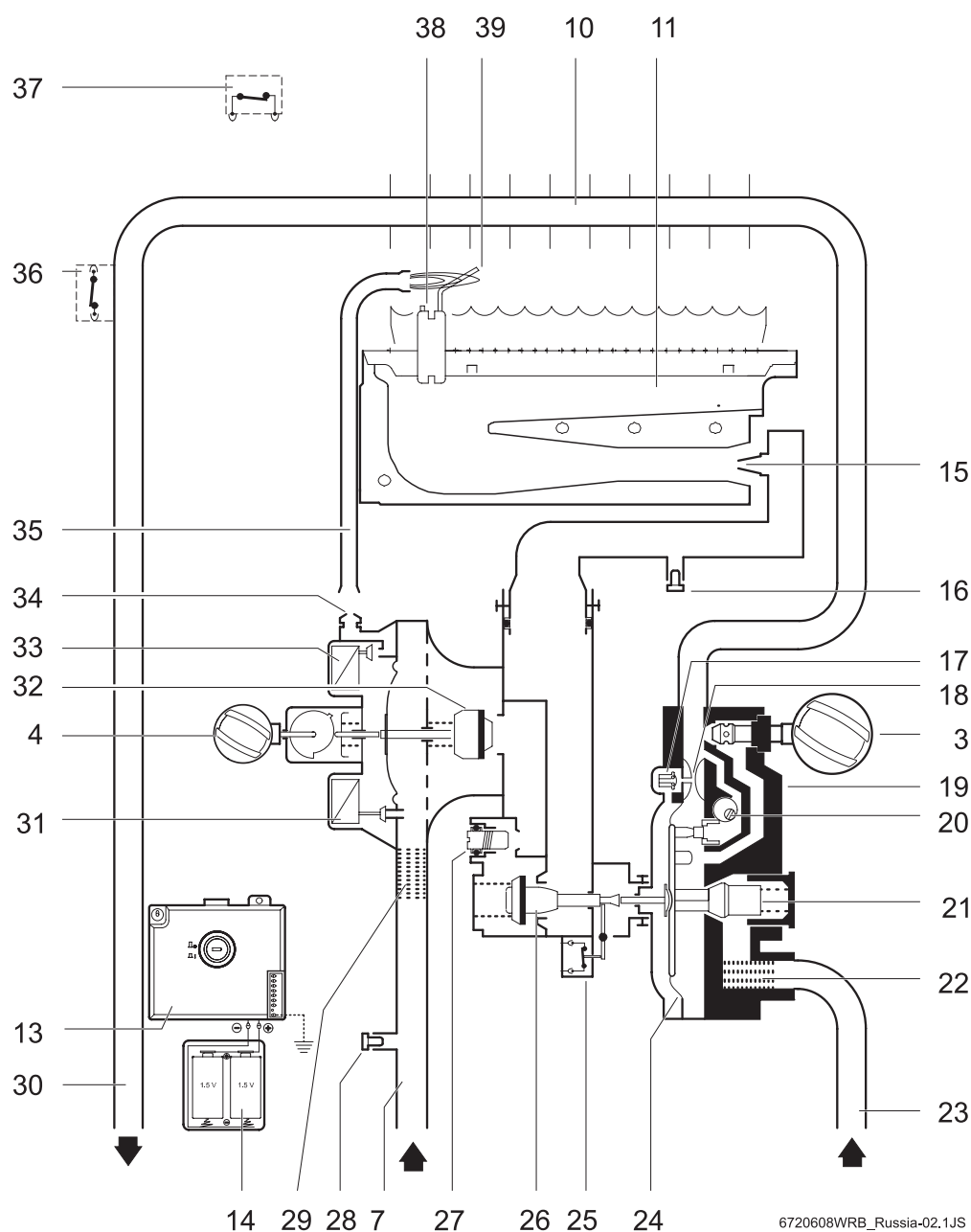
Рис 2 Функциональная схема
