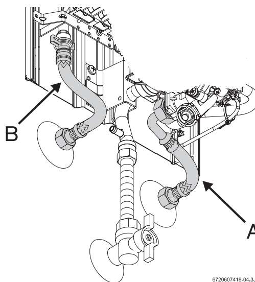
Рис 5 Подключение водопровода
