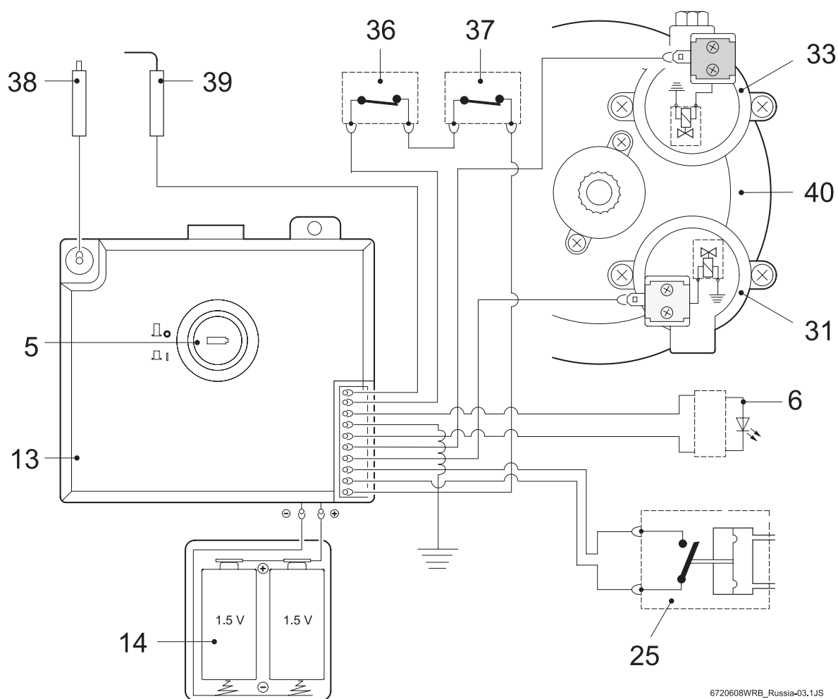
Рис 3 Электросхема
