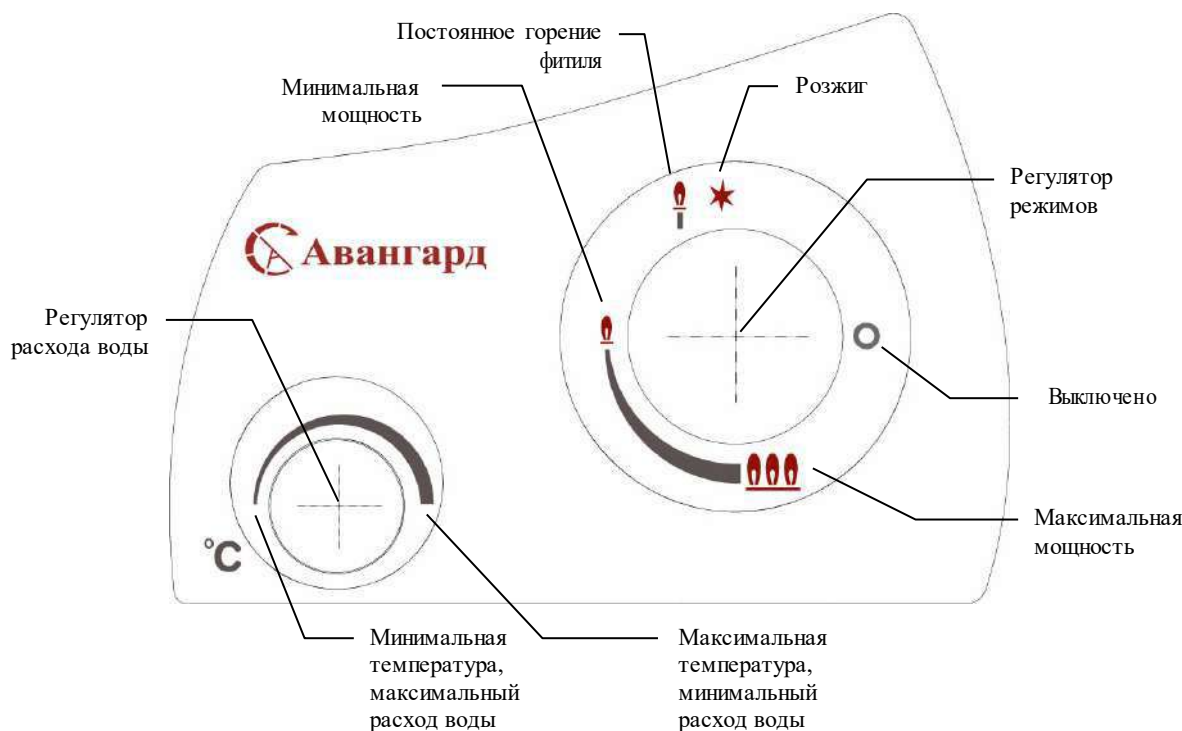
Рисунок 1. Панель управления водонагревателей серий S и SE.
