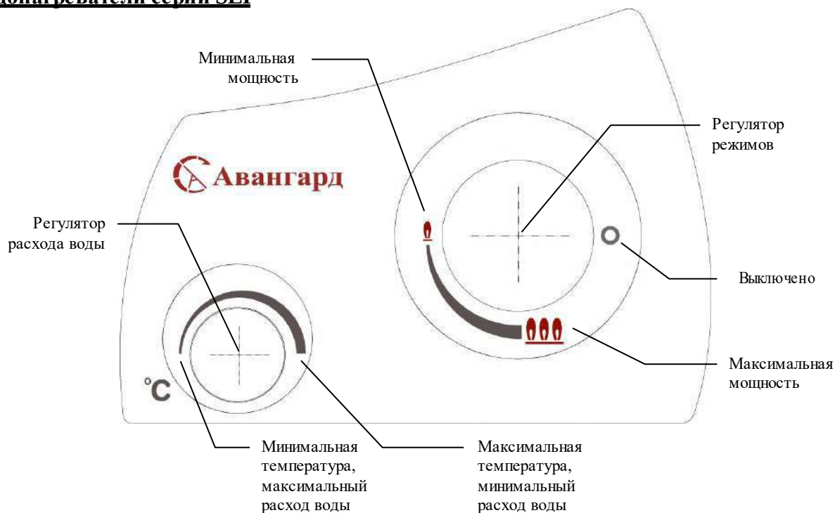
Рисунок 3. Панель управления водонагревателей серий SEI.
