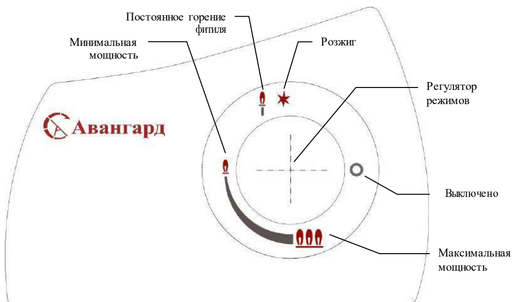
Рисунок 2. Панель управления водонагревателей серии В.
