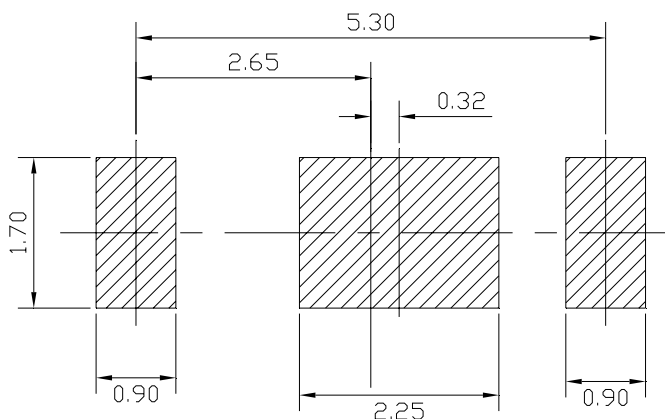
Рекомендуемый размер печатных проводников
